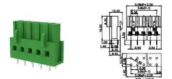
MC-RU5.08SVXX-0001
