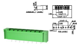
MC-PA5.0HXX-I-0002
