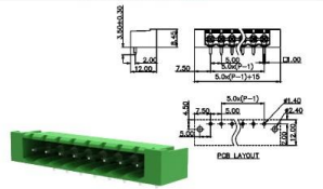
MC-PA5.0HXX-I-0002
